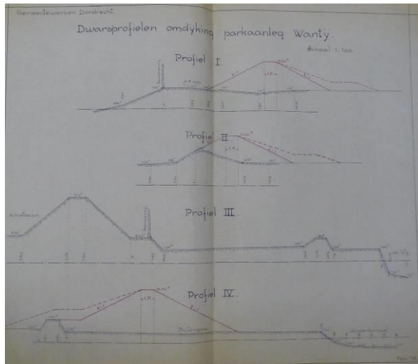
Profielen
